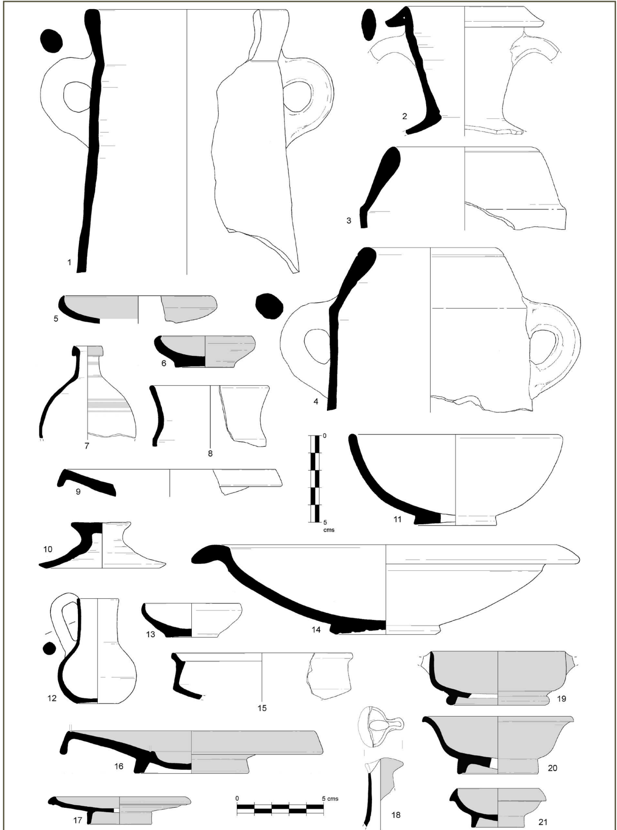
Fig. 4 - Cuadro tipológico de síntesis de algunas de las producciones anfóricas, comunes y barnizadas características de la actividad del alfar de Torre Alta a mediados y segunda mitad del s. -III, según los resultados de las recientes actuaciones en el yacimiento (Sáez, 2004 y 2005).
