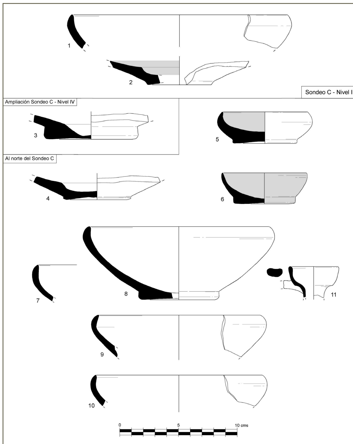
Fig. 3 - Producciones comunes y de barniz rojo de la escombrera documentada en el Sondeo C y su entorno en el alfar de Villa Maruja, en contextos del s. -IV avanzado o inicios del -III.
